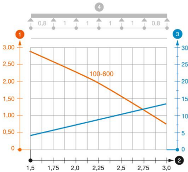
电缆桥架 SKS 85负载图
